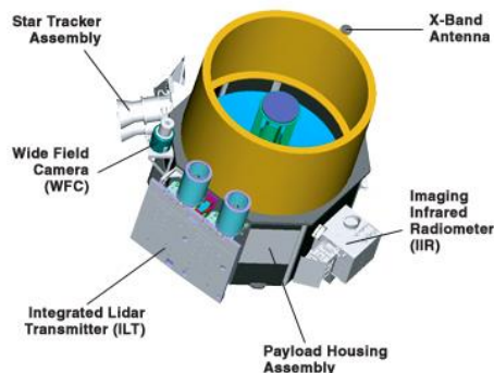
FIG.5. LIDAR – CALIOP [47]
